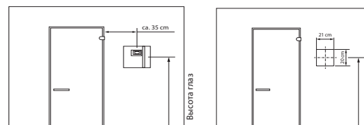
Вырез в стене при монтаже в стене
